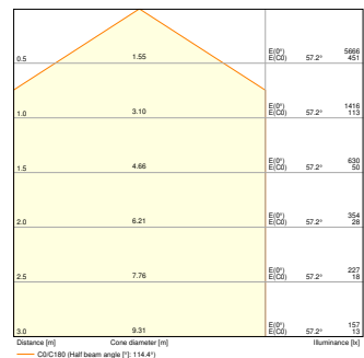
PL SF 674 V 32W 930 4160lm
