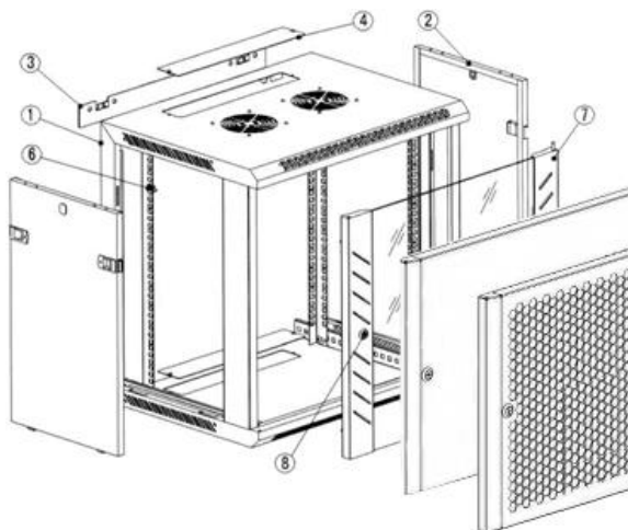
Schéma rozvaděče – dveře sklo, plné a perforované
