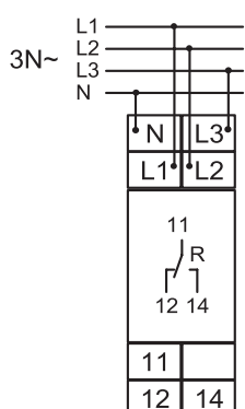
Příklad zapojení relé E1YF
