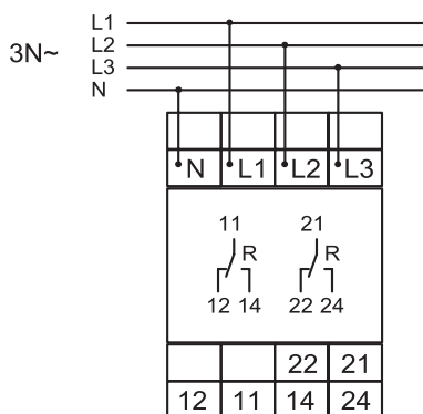
Příklad zapojení relé E3YF
