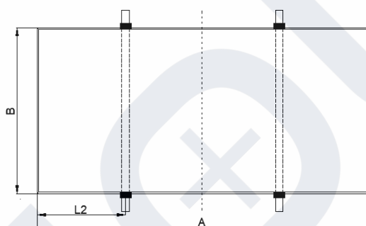
Instalace úpínky s příčným nosníkem (A3) Velikost úpínky \geq 50 mm
