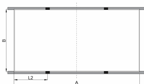
Instalace úpínky bez příčného nosníku (B3) Velikost úpínky \geq 50 mm
