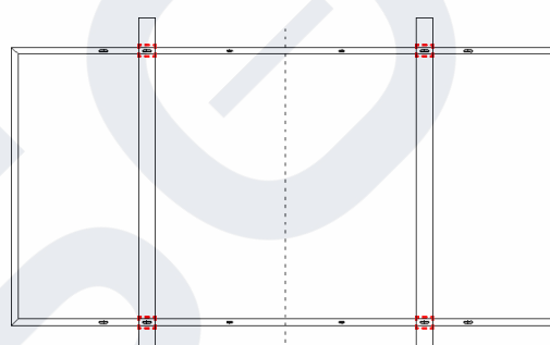
4 vnitřní instalační otvory s příčným nosníkem (A2)
