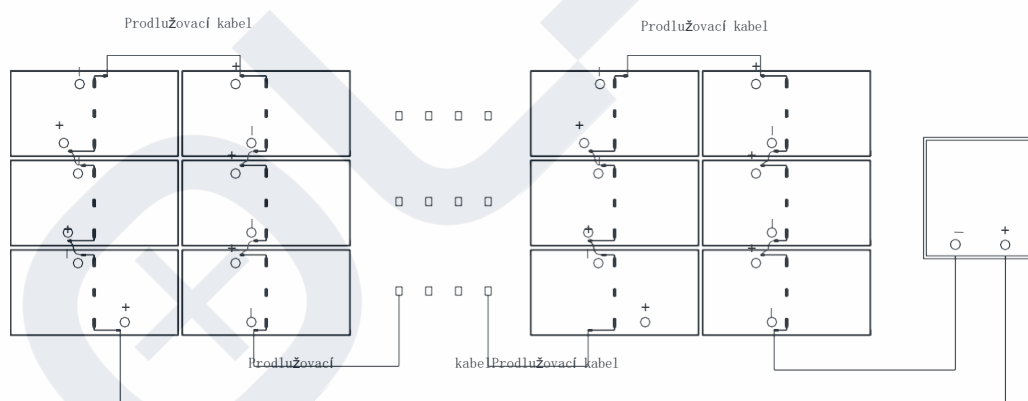
Obr. 9-2 Vodorovná instalac modulů s krátkým kabelem
